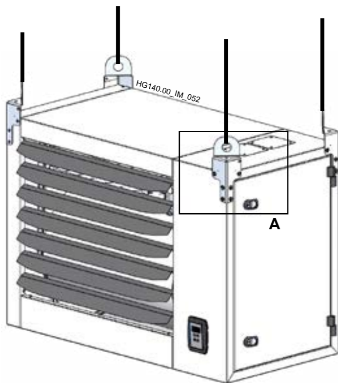
DETAL A: 24 śruby i 24 podkładki zębate stanowiące część wyposażenia zestawu
