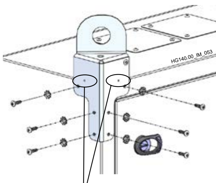
DETAL A: 24 śruby i 24 podkładki zębate stanowiące część wyposażenia zestawu
