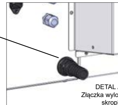
Otwór odprowadzający skropliny
